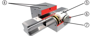
Abb. 2: MK Element im Schnitt
